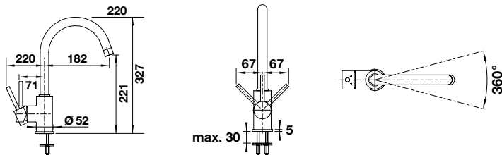
DISEGNI TECNICI
