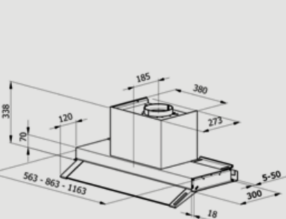
SILENZIO / SILENZIO PLASMA p.145
